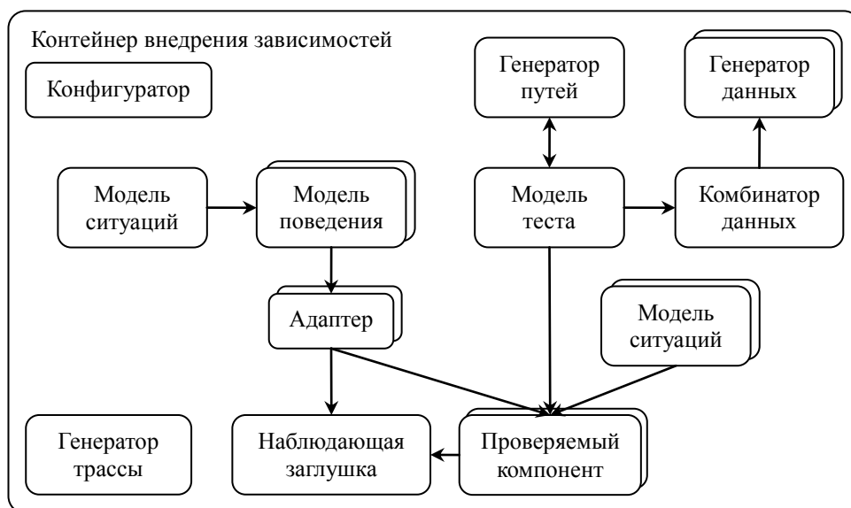
Рисунок 1. Схема построения тестовой системы.
